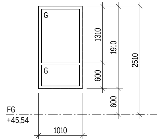
F10d Antal: Enl. tabell 1 Utvändigt fast fönsterparti 2 3-glas isolerruta
