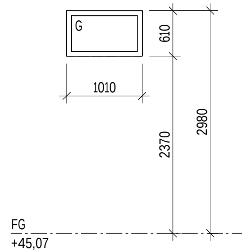
F10a Antal: Enl. tabell 1 Utvändigt fast fönsterparti 2 3-glas isolerruta
