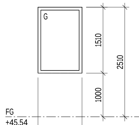
F10h Antal: Enl. tabell 1 Utvändigt fast fönsterparti 2 3-glas isolerruta
