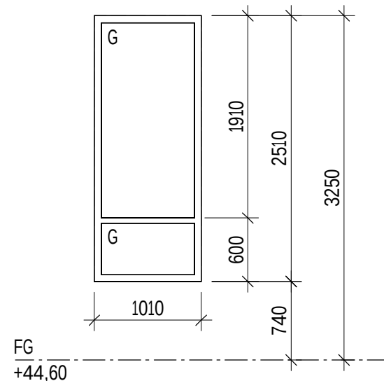
F10i Antal: Enl. tabell 1 Utvändigt fast fönsterparti 2 3-glas isolerruta
