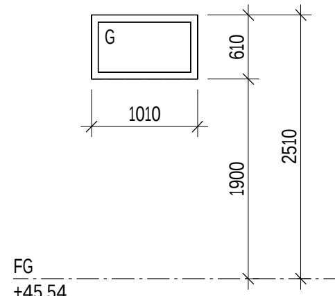
F10c Antal: Enl. tabell 1 Utvändigt fast fönsterparti 2 3-glas isolerruta
