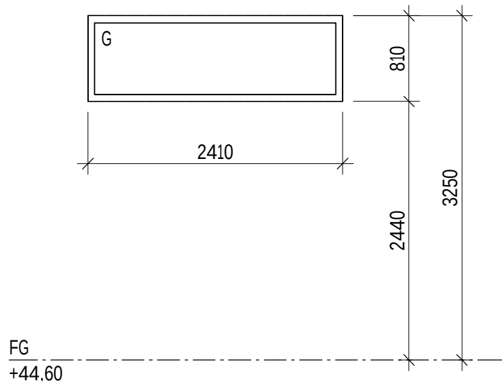
F24a Antal: Enl. tabell 1 Utvändigt fast fönsterparti 2 3-glas isolerruta
