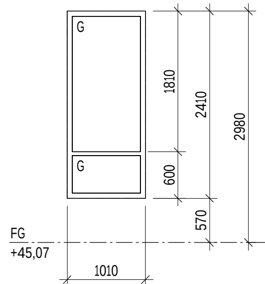
F10b Antal: Enl. tabell 1 Utvändigt fast fönsterparti 2 3-glas isolerruta
