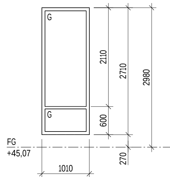
F10f Antal: Enl. tabell 1 Utvändigt fast fönsterparti 2 3-glas isolerruta
